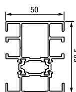
50 mm-es szélesítőprofil
