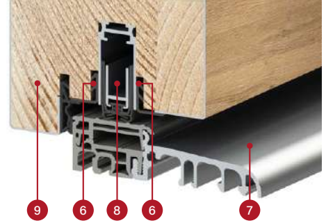
THERMO 78 ajtószárny keresztmetszete takaró tömítéssel és anélkül, alumínium küszöb
