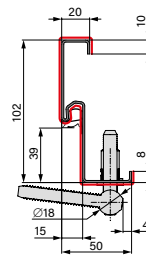
ACÉL SAROK AJTÓTOK
