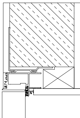
Falcolatlan ajtó vízszintes metszete
