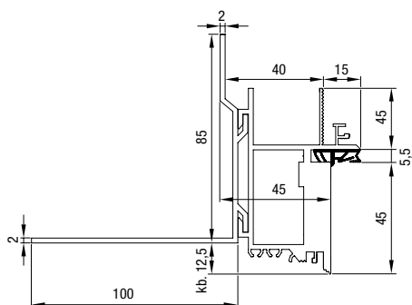
Zeroline tapétaajtó tok méretezése
