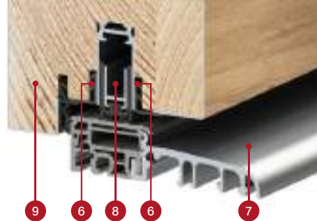
THERMO 78 ajtószárny keresztmetszete takaró tömítéssel és anélkül, alumínium küszöb
